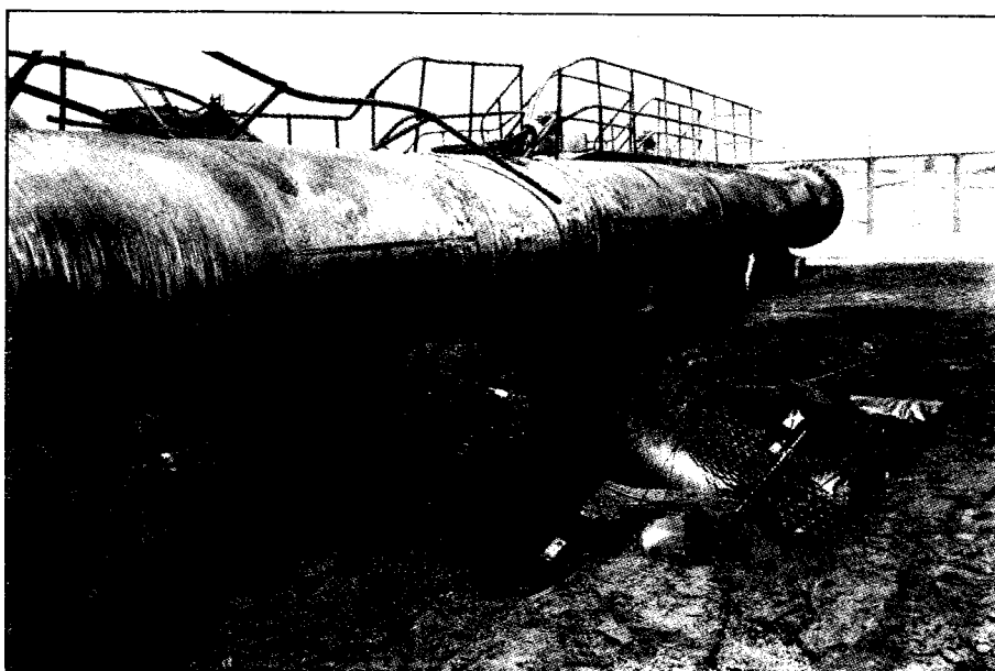
أحد انفجارات أنابيب تجميع النفط
